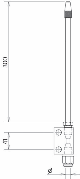
TERMINALI CON UGELLO DECABON DIMENSIONI D'INGOMBRO
