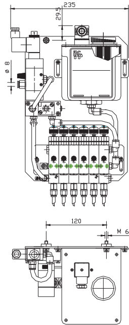
DIMENSIONI D'INGOMBRO AGGF
